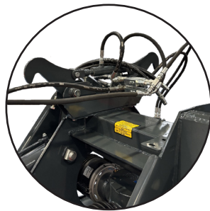
Bloccaggio idraulico Hydraulic locking
