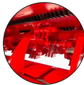
Rotore con martelli rotanti 360° Rotor with 360° rotating hammers
