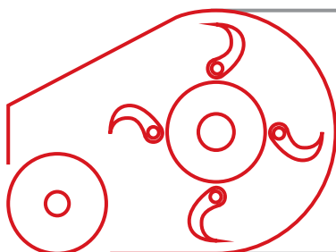
SISTEMA DI TRASPORTO CON 2 RUOTE TRANSPORT SYSTEM WITH 2 WHEELS
