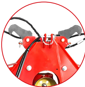
Bloccaggio meccanico Mechanical locking
