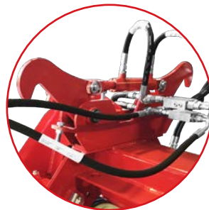
(OPTIONAL) Bloccaggio idraulico Hydraulic locking
